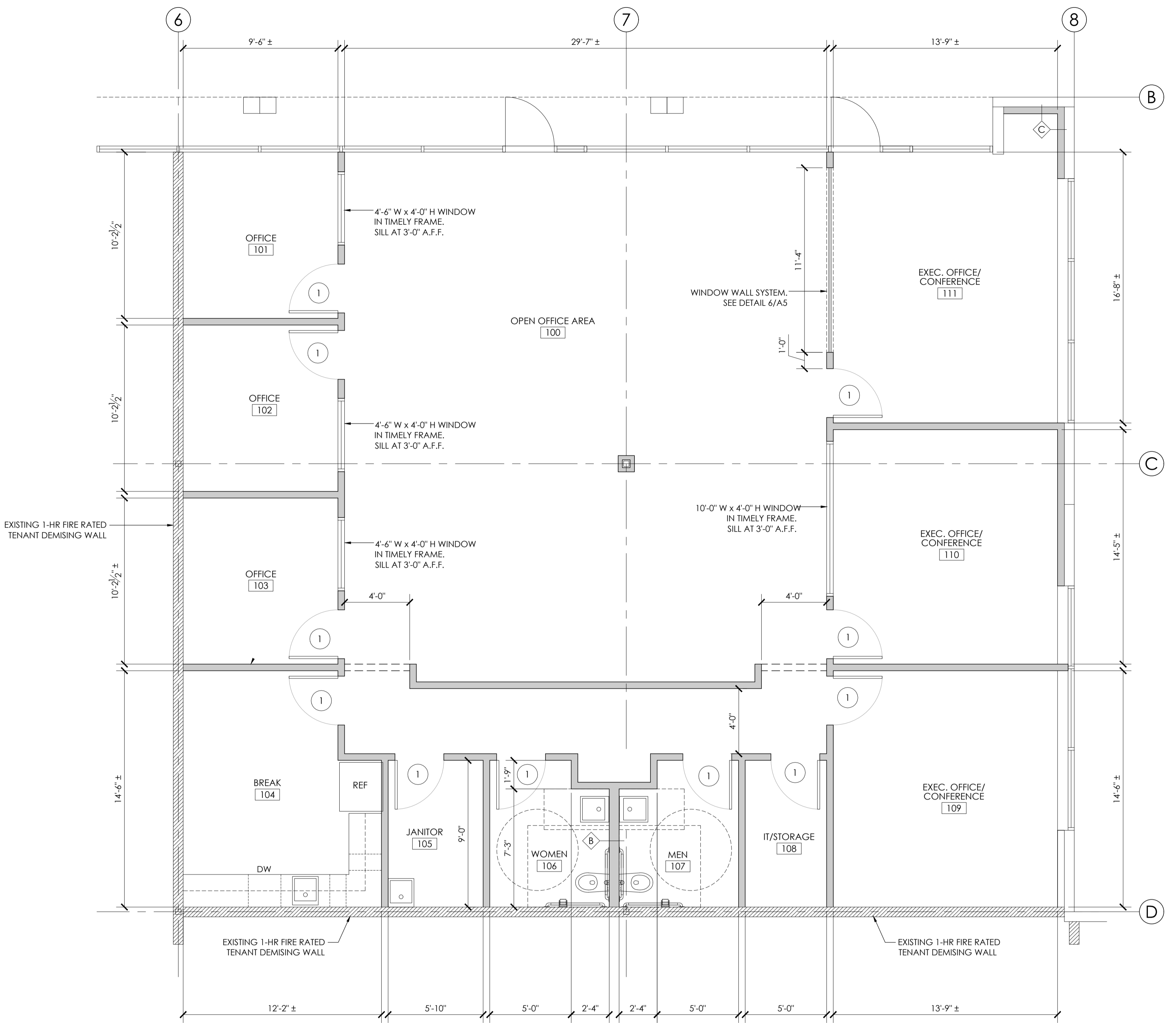
1 Floor Plan Scale: 1/8" = 1'-0"
